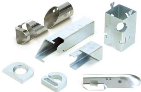
丸パイプ/角パイプ. 3次元レーザー加工
